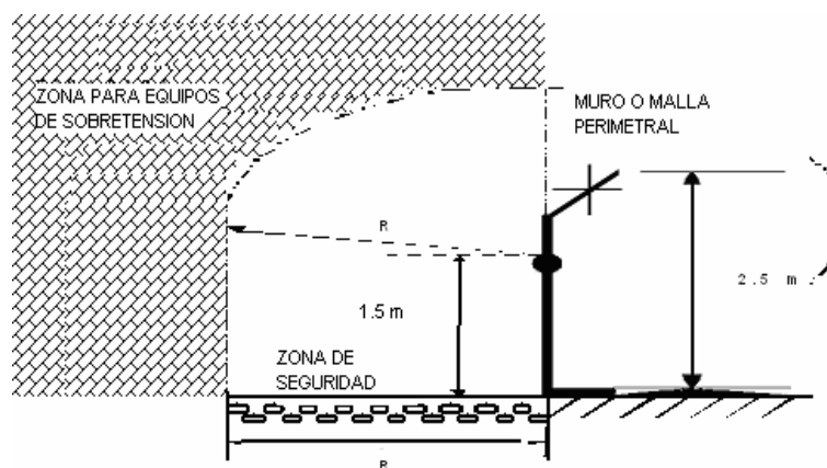
Figura 22. Distancias de seguridad para prevenir contactos directos en subestaciones exteriores.
