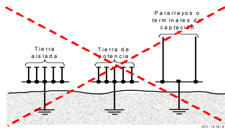
Figura 12. Puestas a tierra separadas o independientes
