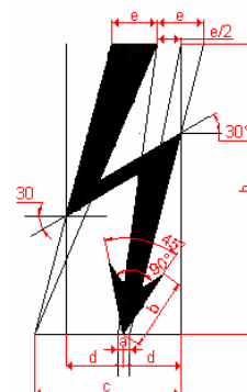
Figura 4. Símbolo de riesgo eléctrico
