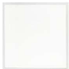
Panel 30x30 26W Luz Blanca / Fresca 35.000 H 2.340 lm 110-240 V
